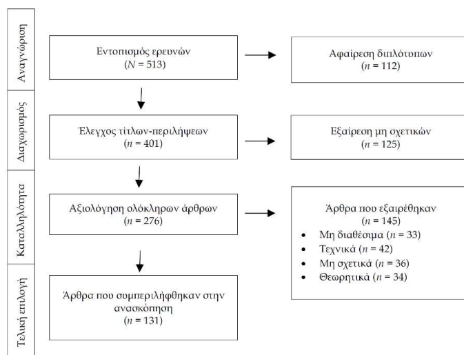
Σχήμα 1. Διάγραμμα ροής της μεθοδολογίας PRISMA
