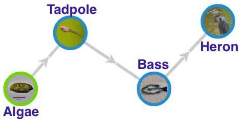
Εικόνα 6. Ροή της ενέργειας μεταξύ των οργανισμών (foodweb)
