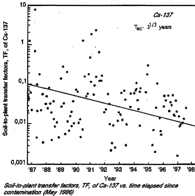
Διάγραμμα 1. Παράγοντας μεταφοράς, TF, από το χώμα στο γρασίδι για το ^{137}\text{Cs} συναρτήσει του χρόνου
