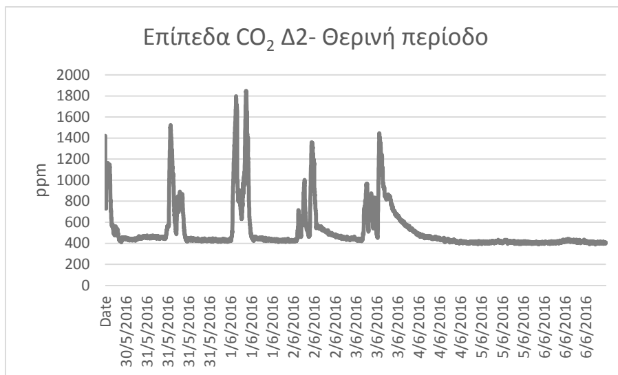
Εικόνα 19: Επίπεδα διοξειδίου του άνθρακα αίθουσας Δ2 θερμής περιόδου
