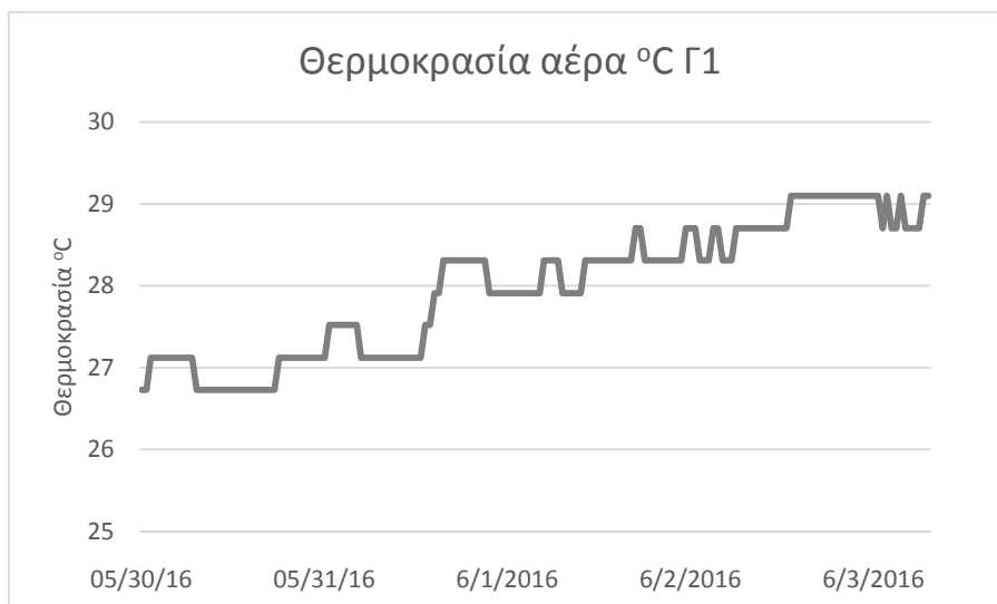
Εικόνα 8: Θερμοκρασία αέρα θερινής περιόδου αίθουσας Γ1
