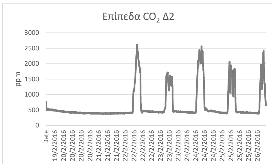
Εικόνα 18: Επίπεδα διοξειδίου του άνθρακα αίθουσας Δ2
