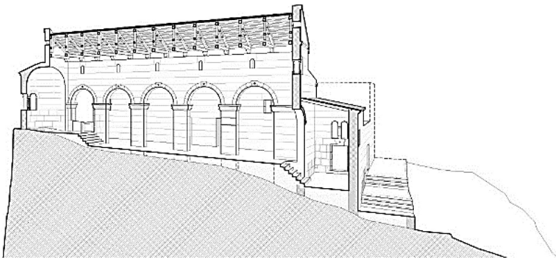
Προοπτική τομή από βόρεια της ιουστινιάνειας βασιλικής της Αγίας Κορυφής.
