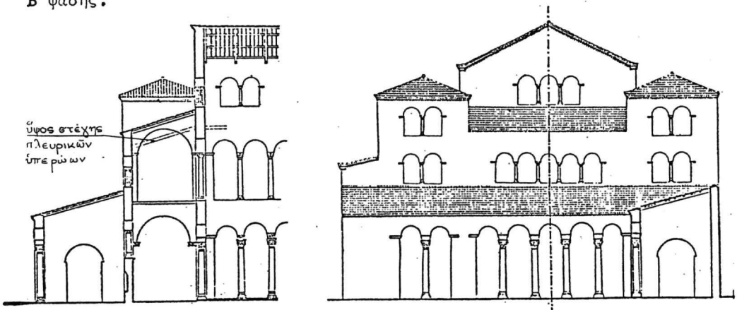
Σχ. 1. ΑΠΟΚΑΤΑΣΤΑΣΗ ΔΥΤΙΚΗΣ ΠΛΕΥΡΑΣ, ΤΟΜΗ Β ΟΨΗ
