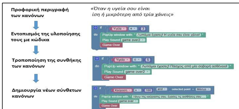
Εικόνα 3: Η προοδευτική χρήση της δομής επιλογής κατά την διασκευή κανόνων στο ChaiCo
