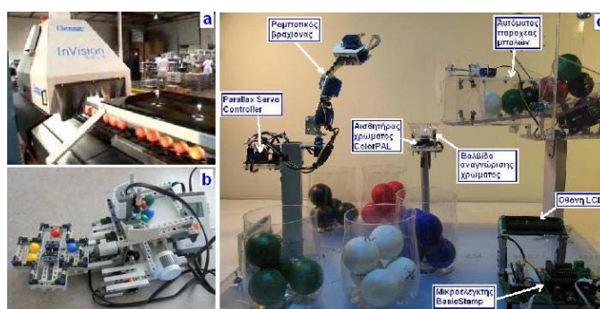
Σχήμα 1. (a) Βιομηχανικός ΧΤ φρούτων, (b) ΧΤ με το πακέτο Lego NXT , (c) ΧΤ με χρήση του Parallax microcontroller
