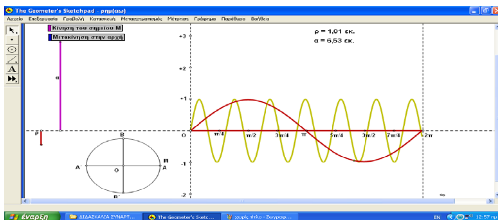
Σχήμα 3: οι γραφικές παραστάσεις των συναρτήσεων f(x)=\eta\mu x και f(x)=\rho\eta\mu(\alpha x)
