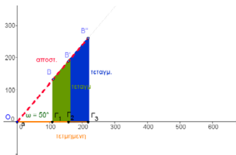
Σχήμα 2 Όμοια τρίγωνα
