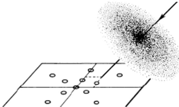
Σχήμα 2. Ο δίσκος σωματιδίων του ατμοσφαιρικού καταιονισμού.
