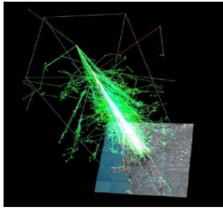
Σχήμα 1. Μια καλλιτεχνική απεικόνιση ενός ατμοσφαιρικού καταιονισμού πάνω από μια πόλη.
